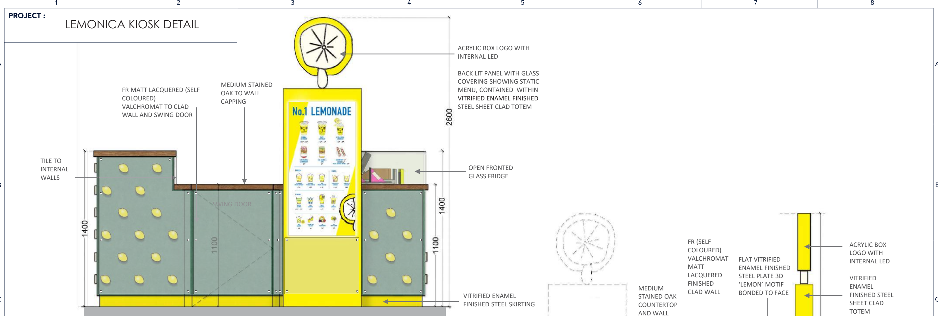
ELEVATION BB
